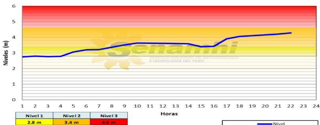
NIVELES HORARIOS DEL RÍO HUALLAGA ESTACIÓN TINGO MARÍA
